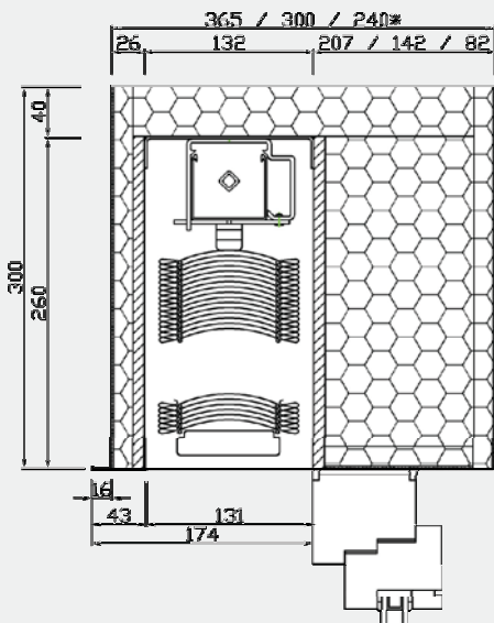
Jalousiekasten Iso
