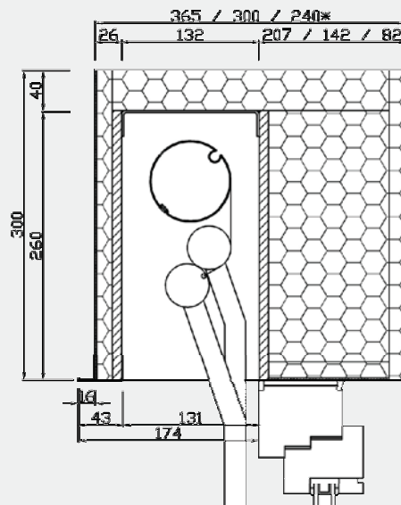
Markisenkasten Iso
