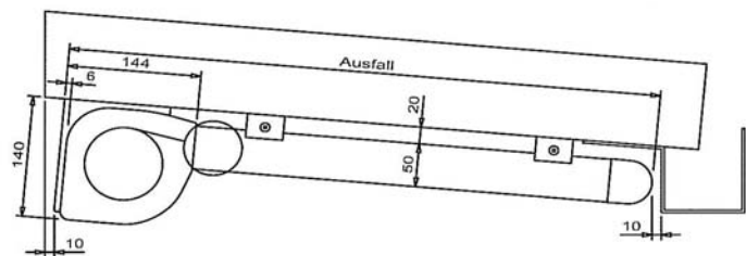
Ansicht von unten
